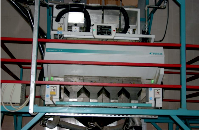
Şekil 7. Sorteks Makinası
