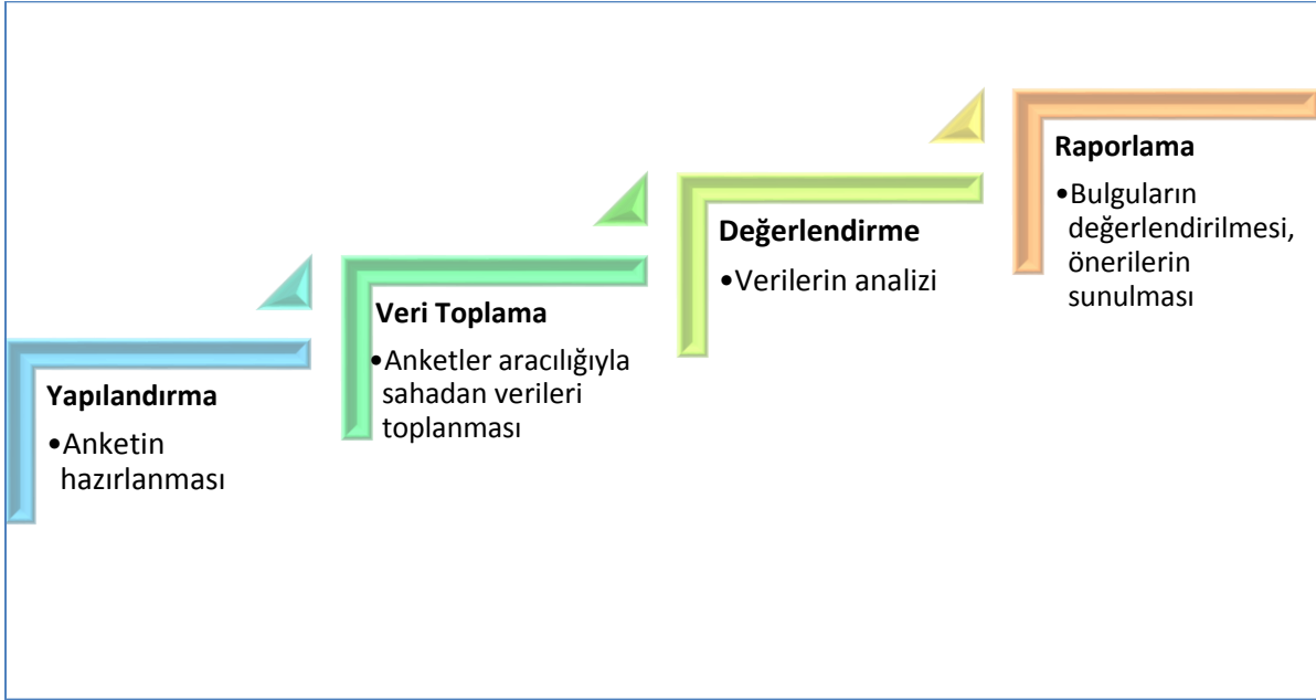
Şekil 1: Değerlendirme Metodolojisi
