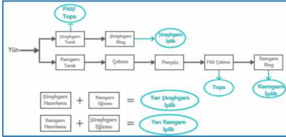
Şema 2: Kamgarn/Ştrayhgarn veya Yarı Kamgarn/Yarı Ştrayhgarn İplik
