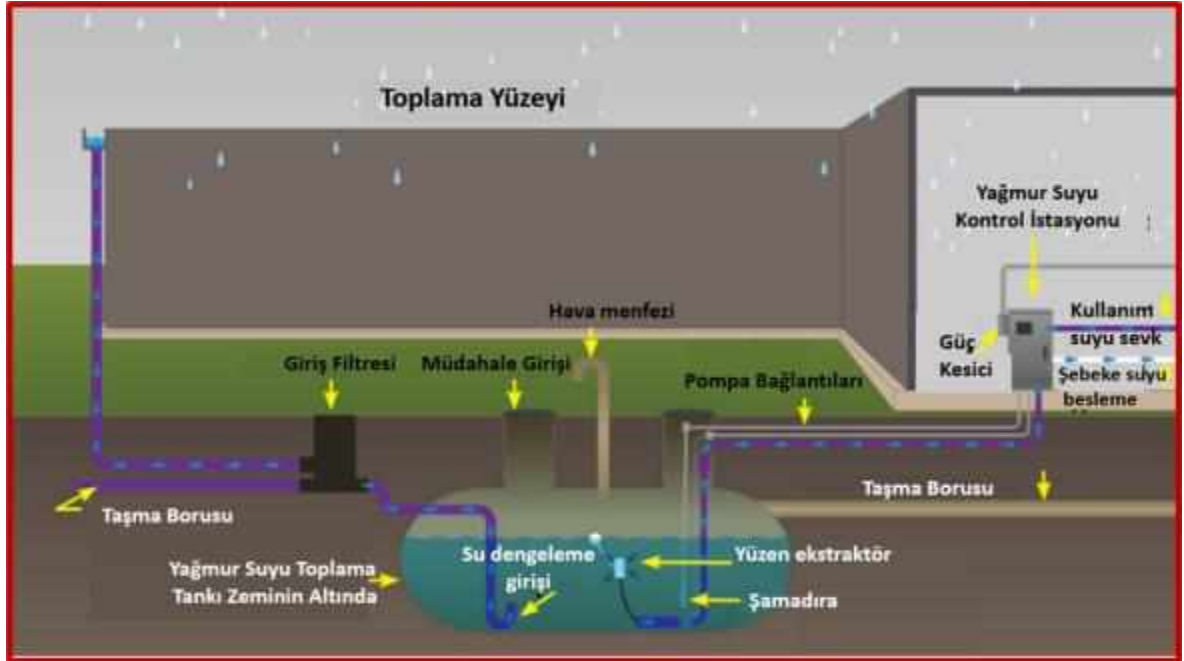
Şema 7: Yağmur Suyu Toplama Sistemi
